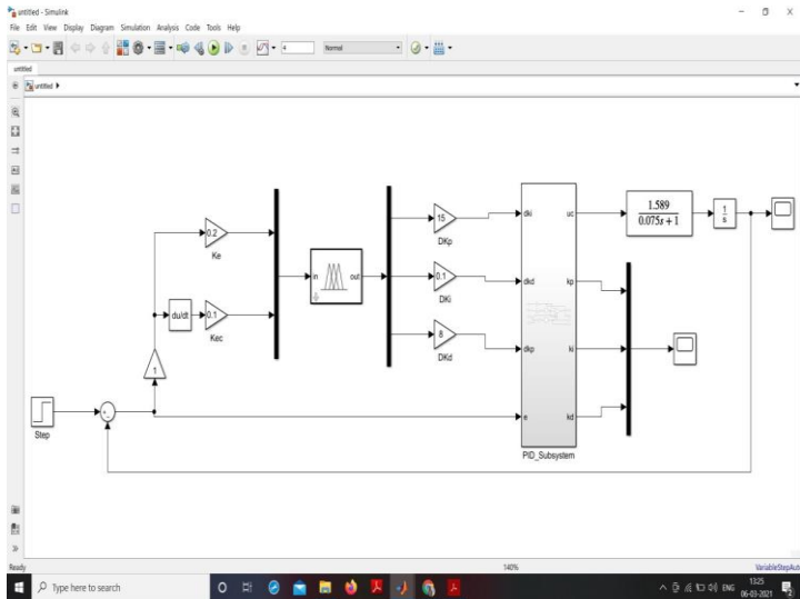
Fig. 4: Simulink Model
